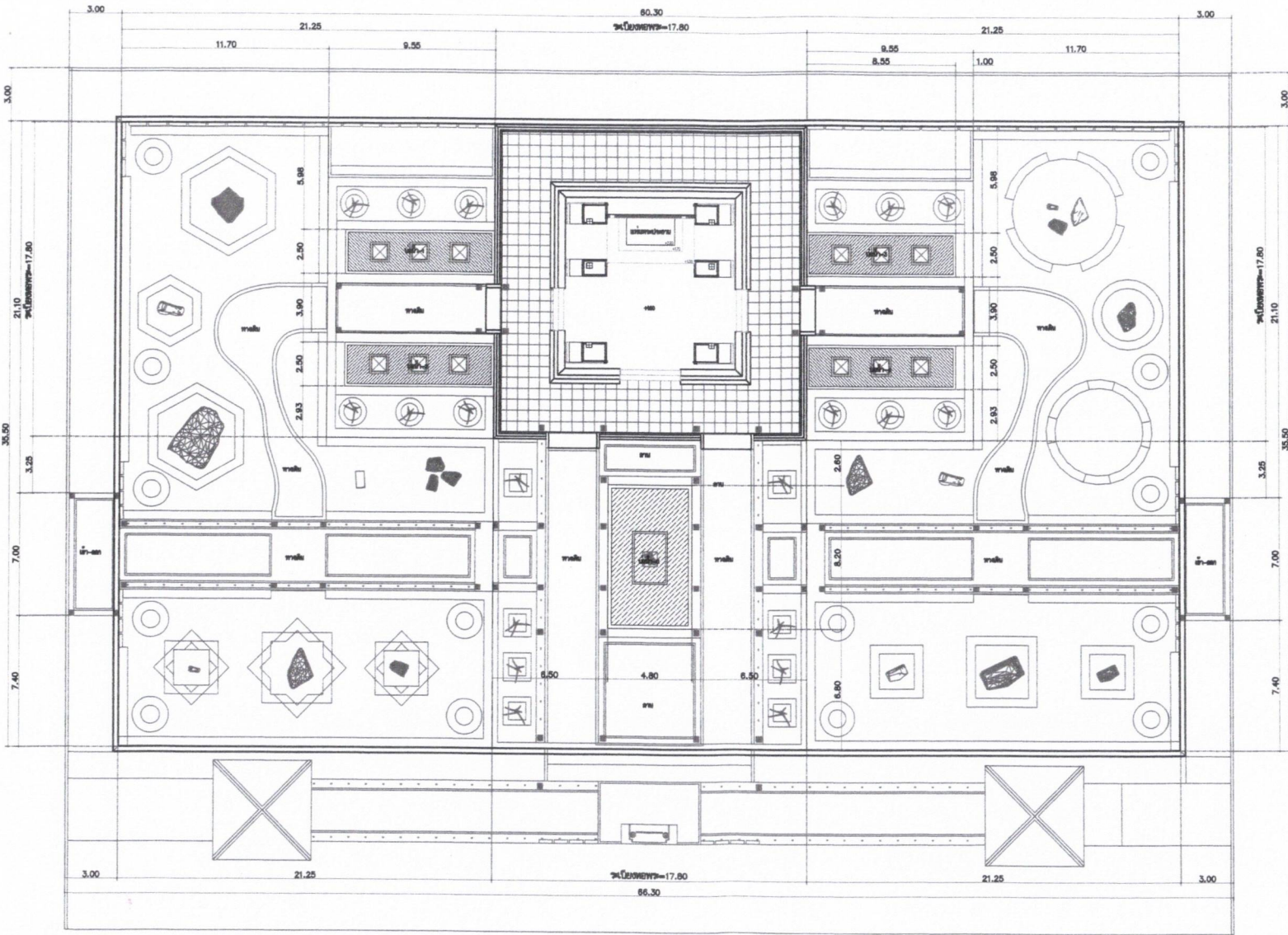
แปลนแสดงตำแหน่งบ่อน้ำ Scale: 1:100
