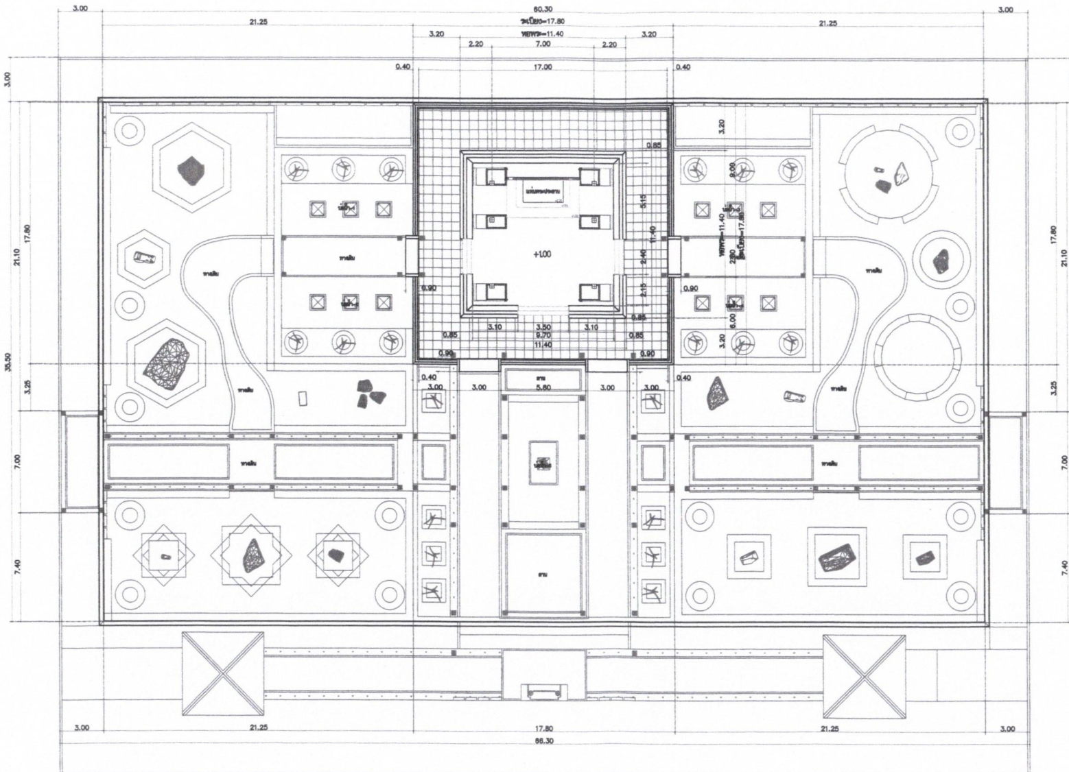
แปลนแสดงตำแหน่งศาลาประดิษฐานพระพุทธรูป Scale/1:100
